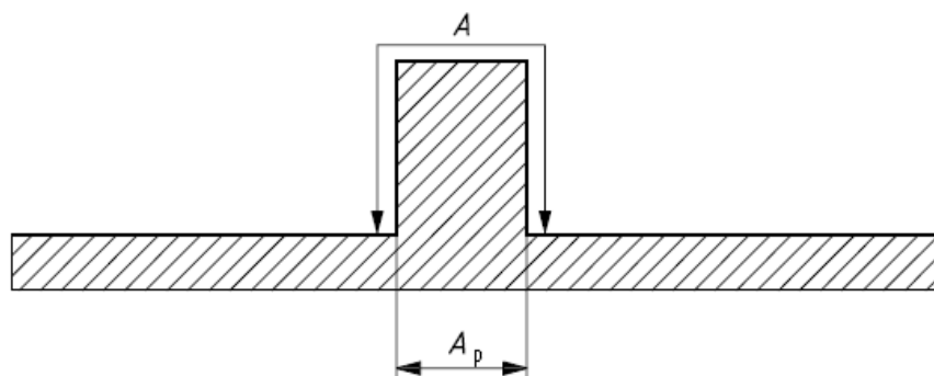
Slika 3.A.1 – Stvarna i projicirana ploština
